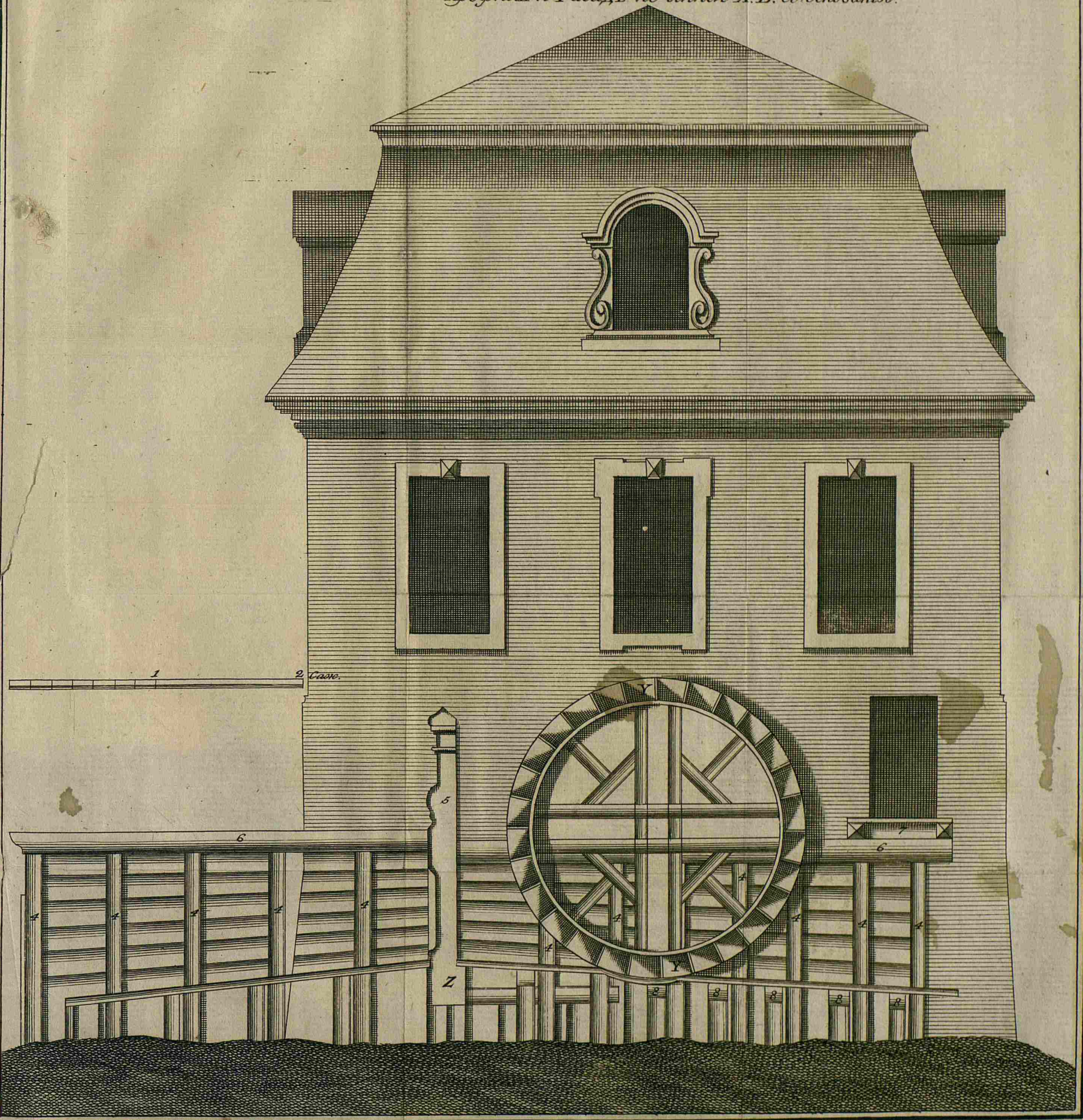
Профиль и Фасадъ по линіи А. В. со основаніи.
