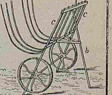
Ч.10. Работная талка Хюгеса (Hughes) для связываемого хлѣба.
