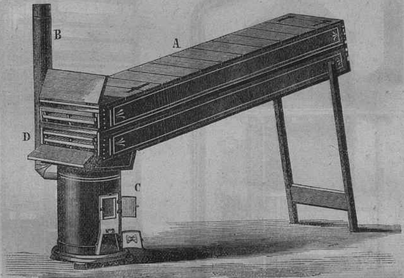
Фиг. 5. Плодосушилка «а мериганга» Ридера.
