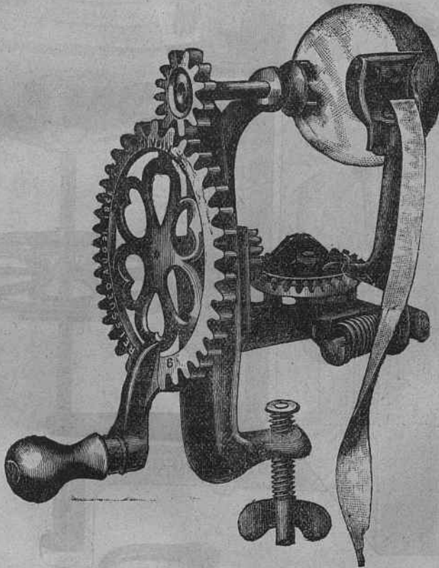
Фиг. 6. Кожицеснимательница «Gold Medal».
