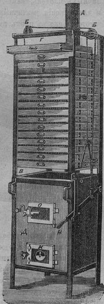
Фиг. 4. Плодосушилка Рера.
