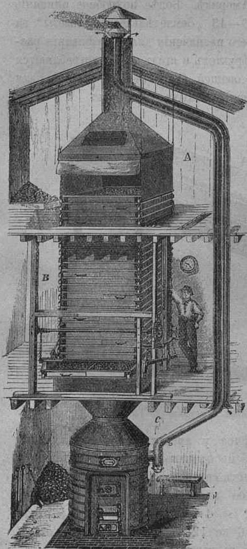
Фиг. 3. Плодосушилки Рейнольда.
