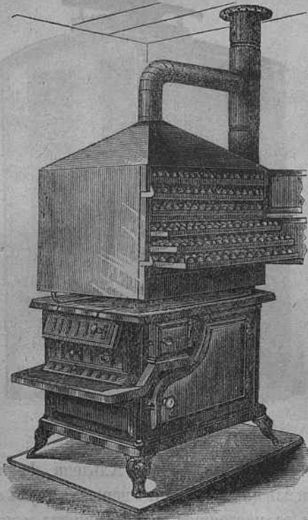
Фиг. 1. Сушильный шкафъ для плиты.
