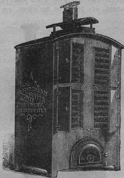
Фиг. 2. Плодосушилка Циммермана.
