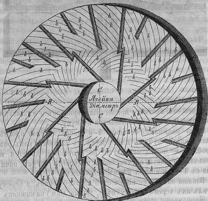
а—чеканка. б—насычка. в—диаметръ. с—ячейка жернова.
