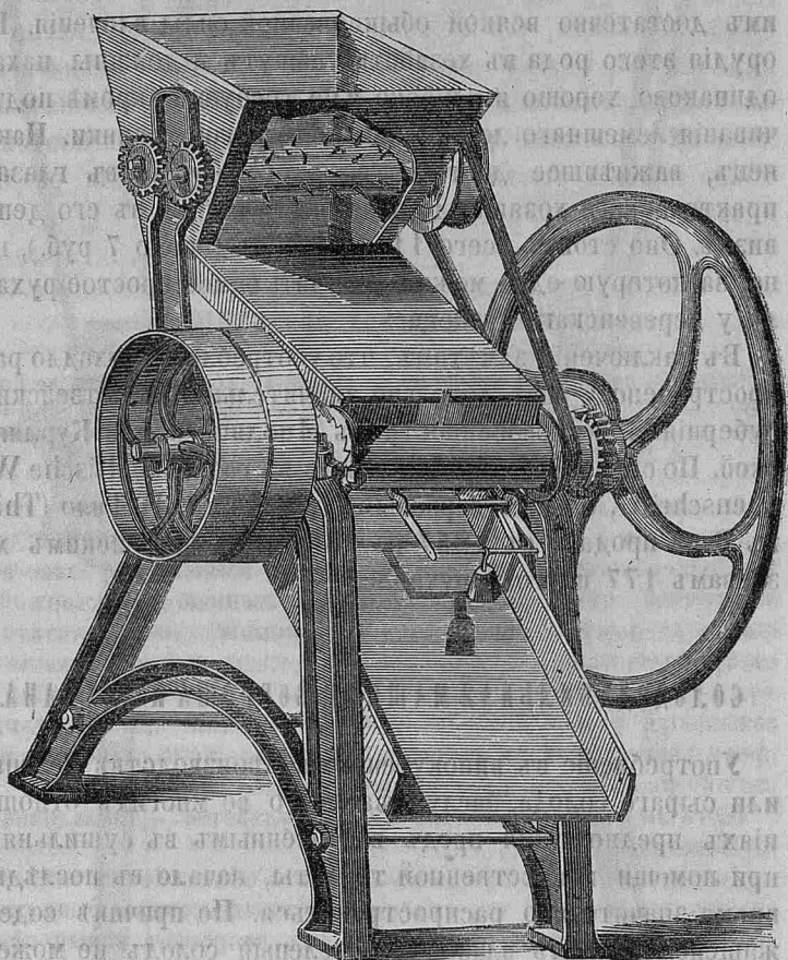
Солодовильная машина Эйхмана.
