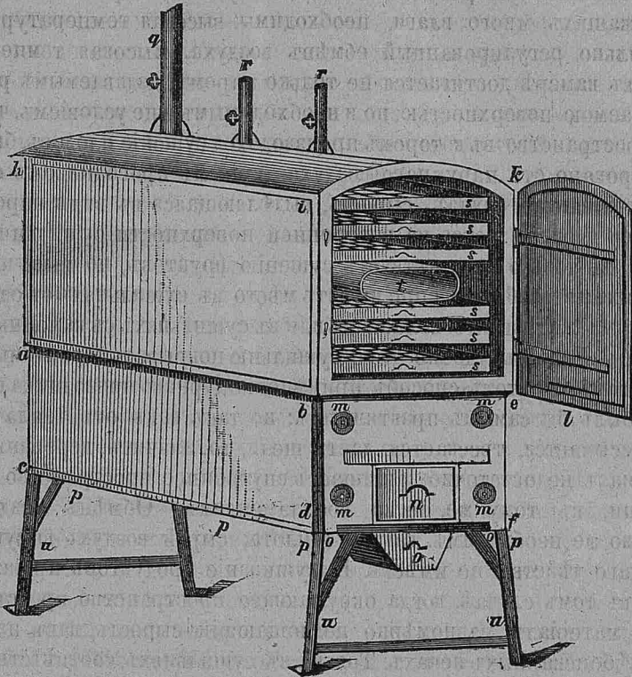
Сушильня для фруктовъ.
