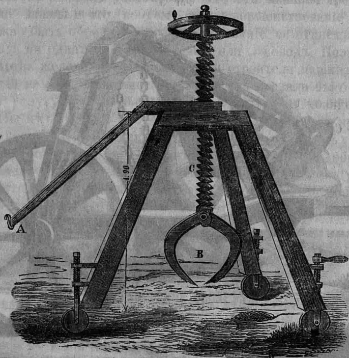
Венгерская корчевальная машина.
