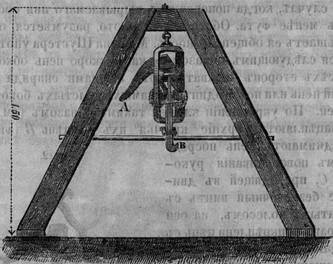
Вюртембергская машина для корчеванія пней.
