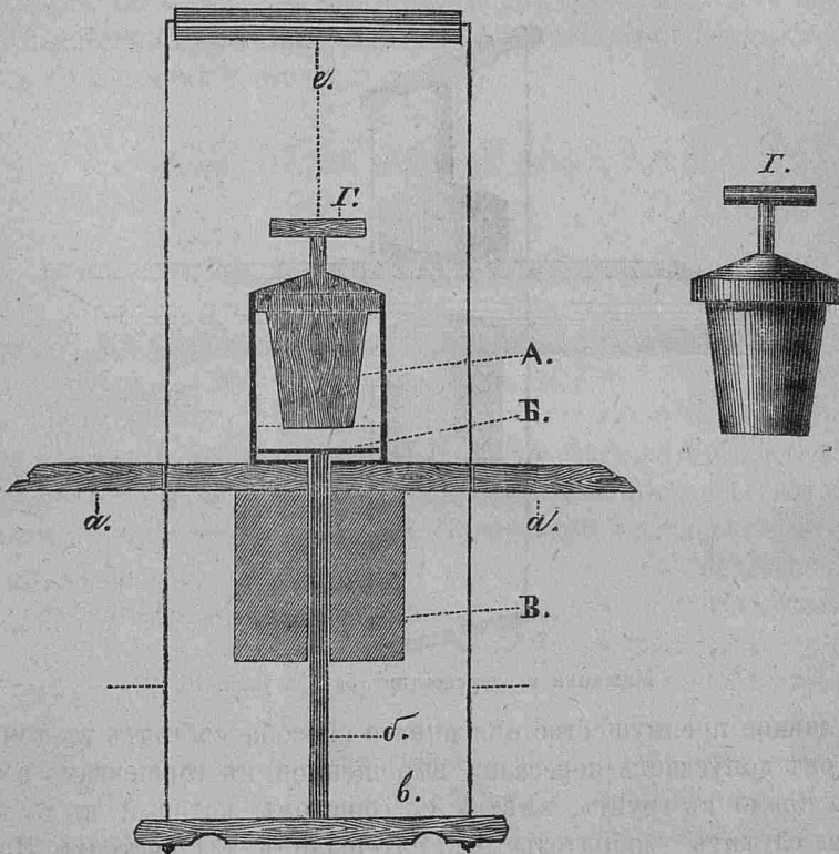
Машинка въ разрѣзѣ.
