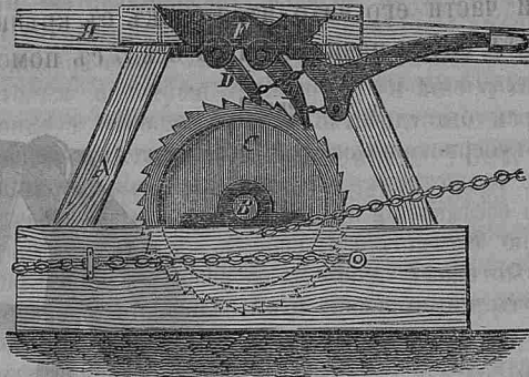
Храповое зацѣпленіе въ корчевальномъ снарядѣ Гоуэ.
