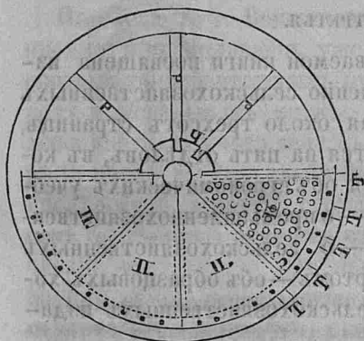
Фиг. 8. Планъ сушильнаго круга.
