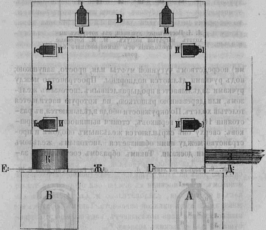
Фиг. 4. Планъ печи, борова и трубы.
