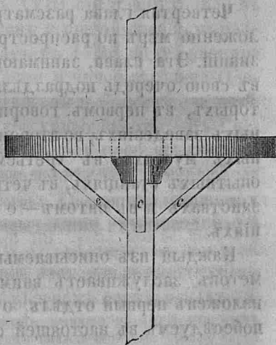
Фиг. 9 показываетъ устройство подпорникъ къ ручкамъ и муфты.
