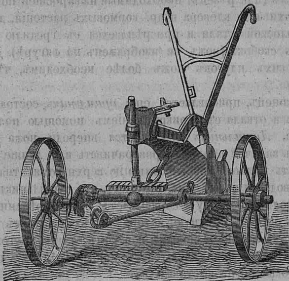
Передковый плугъ Эккерта.
