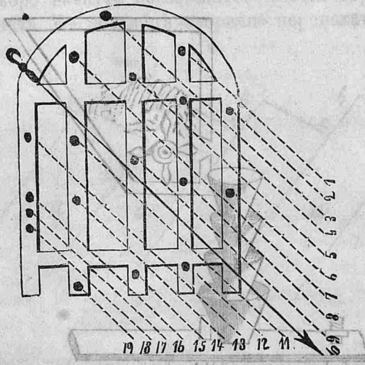
Улучшенная борона.
